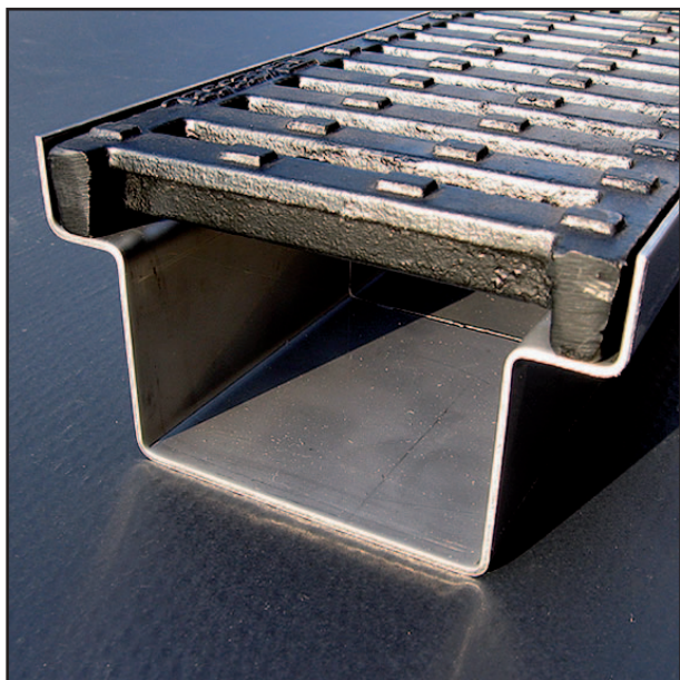
Entwässerungsrinne ERH - Basisform mit Gussrost
