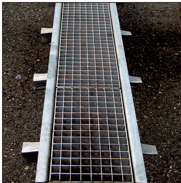
Entwässerungsrinne ERH - Mit Betonierschlaudern und Gitterrost
