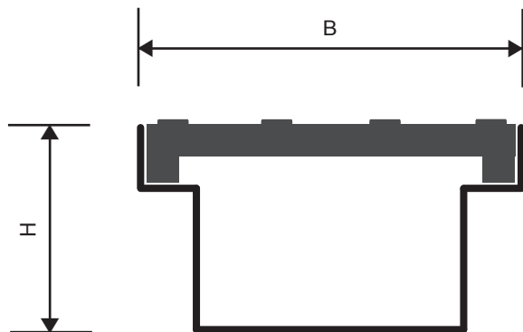
Entwässerungsrinne ERH - Basisform mit Gussrost
