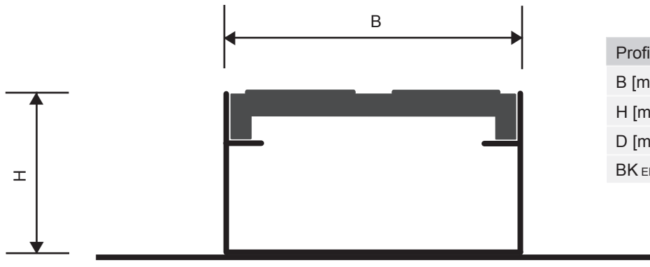
Entwässerungsrinne ER - Basisform mit Gussrost
