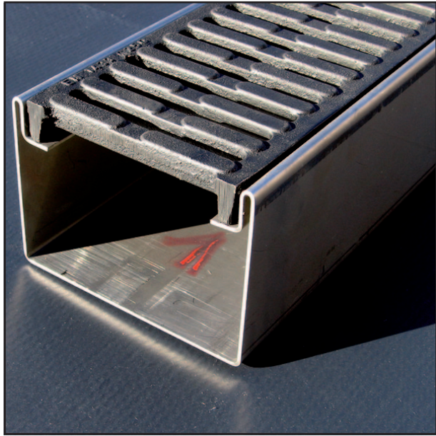
Entwässerungsrinne ER - Basisform mit Gussrost
