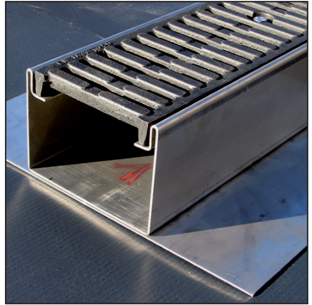
Entwässerungsrinne ER - Mit Abdichtungsflansch und Gussrost
